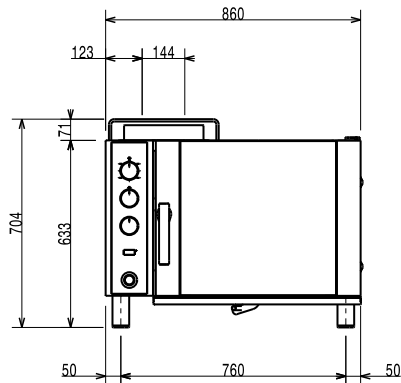
Front aanzicht
